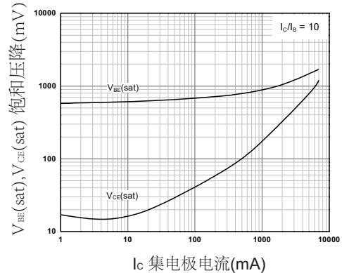
图2. B-E饱和压降,C-E饱和压降
