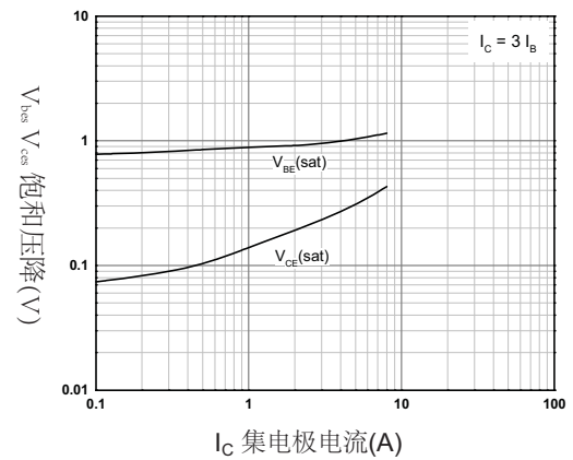
图2 饱和压降
