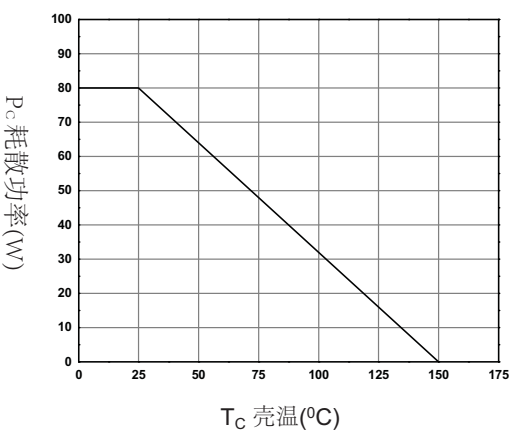
图8 额定功率
