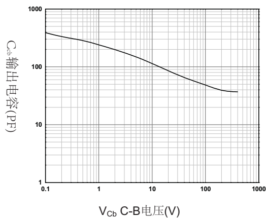
图3 输出电容
