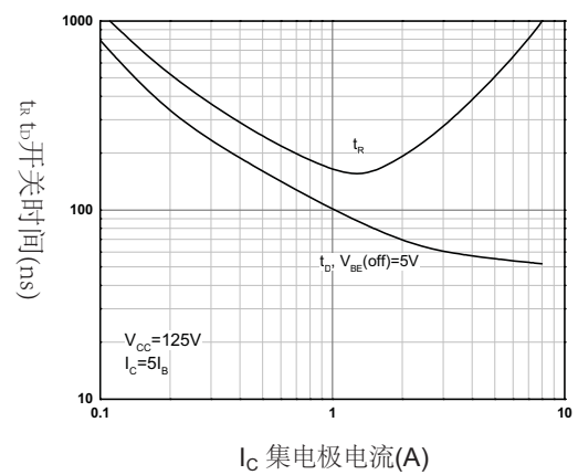
图4 开通时间
