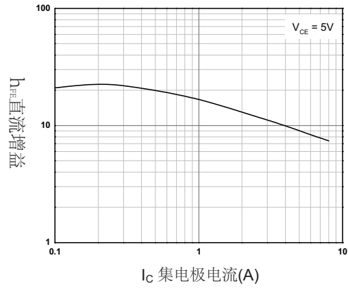
图1.直流增益
