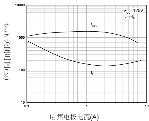
图5 关闭时间
