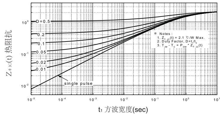
图11-2. 热阻抗变化曲线(TO-220F)
