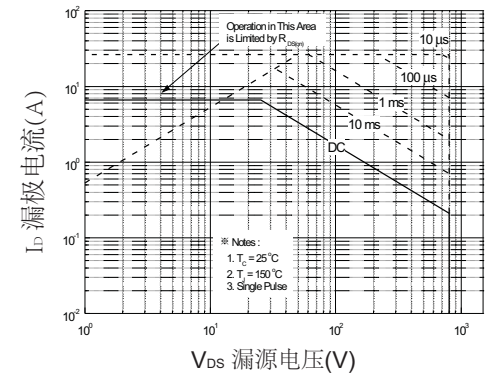
图9-1. 最大安全使用范围(TO-220)
