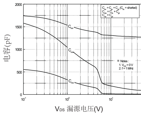
图5. 电容特性
