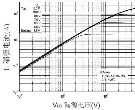
图1. 通态特性
