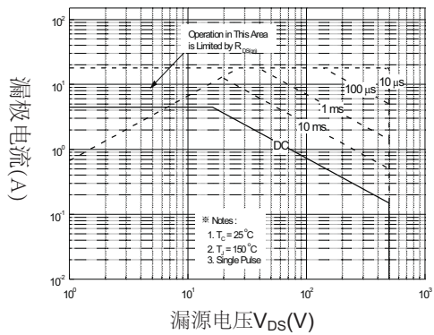
图9-1 FHP730 安全使用范围
