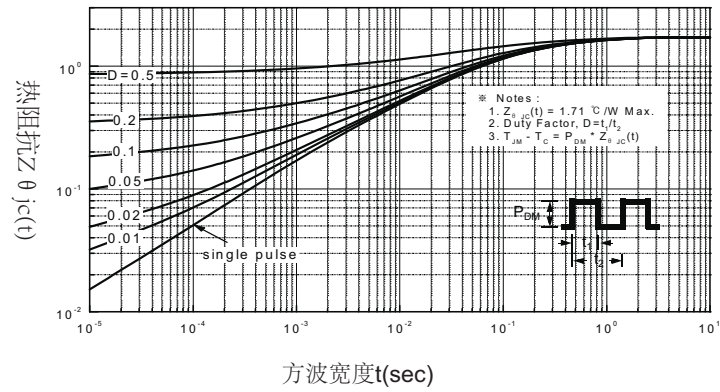
图11-1 FHP730 热阻抗变化
