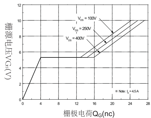
图6 栅极充电荷特性
