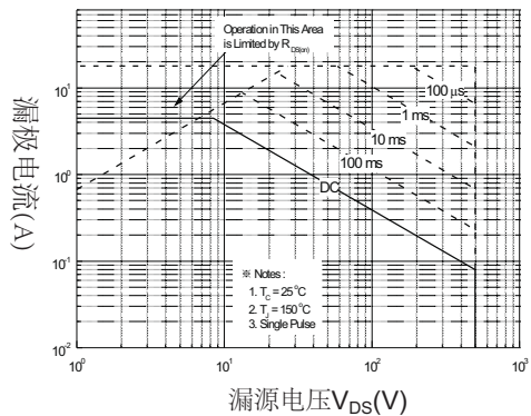
图9-2 FHF730 安全使用范围
